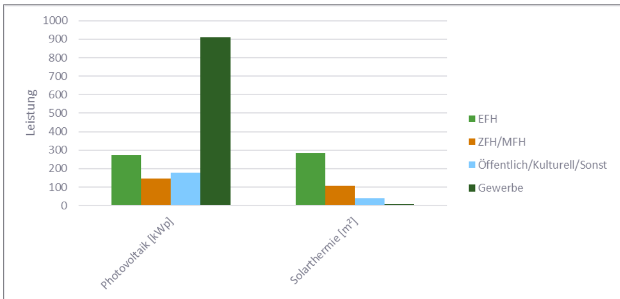
Abbildung 31: Installierte Leistungen Photovoltaik- und Solarthermieanlagen
