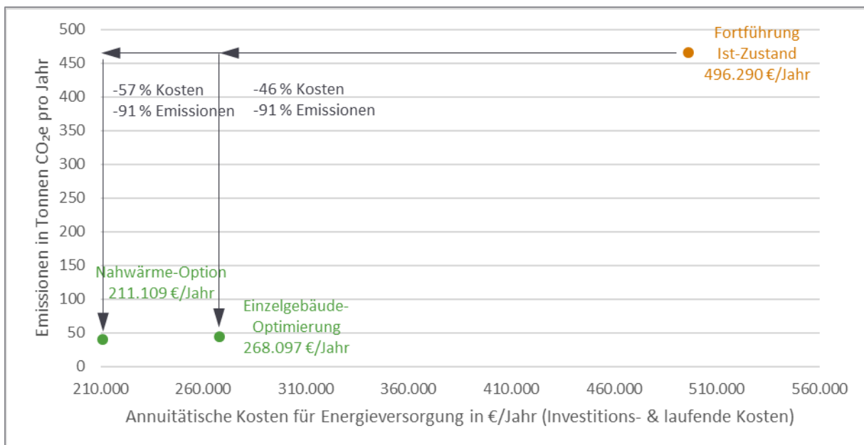
Abbildung 49: Annuitätische Kosten und Emissionen Nahwärmenetz 1, Wetzkeil
